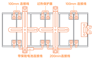
电池连接线 及 压条示意图
