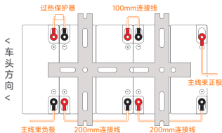
电池连接线示意图
