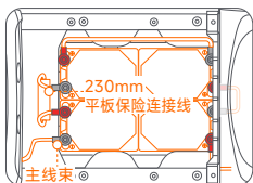
电池链接示意图
