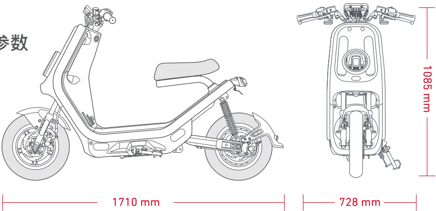
TDR154Z 整车主要技术参数
