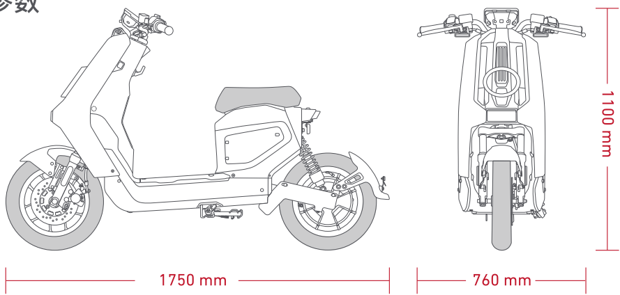
TDR179Z 整车主要技术参数
