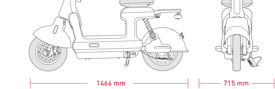
TDR187Z 整车主要技术参数
